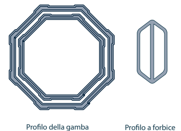
Profilo della gamba
